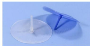
伞形直径：39mm 阀杆直径：2.4mm 扣柱高度：2mm
