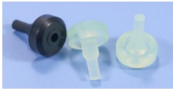
伞形直径：11.6mm 阀杆直径：4.5mm 扣柱高度：4.6mm
