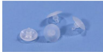
伞形直径：7.4mm 阀杆直径：2mm 扣柱高度：0.9mm
