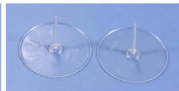
伞形直径：36mm 阀杆直径：1.7mm 扣柱高度：1.5mm
